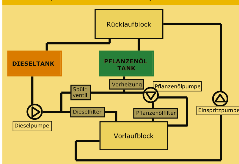
Umrüstkonzept der Firma Graml - Zweitanksystem
