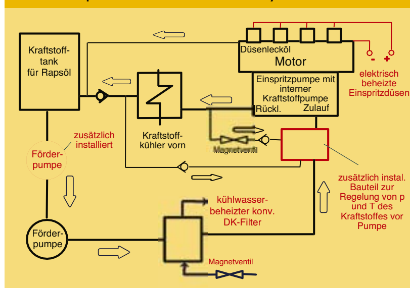
Umrüstkonzept der Firma Hausmann - Eintanksystem
